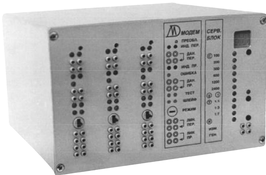
Трехканальный комплекс совмещенной передачи речи и данных ТФМ–3М/ЗДЗС для работы на базе трех одноканальных плат Мультимодема-100/2400 (исполнение ГР) с сервисным блоком
